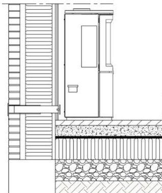
Eksempel på gennemførelse i væg
