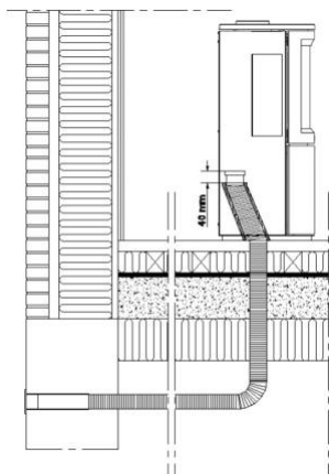
Eksempel på gennemførelse i krybekælder
